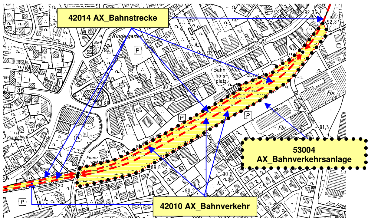
Abbildung 5.4 – 25.: Modellierung mehrerer Bahnstrecken
