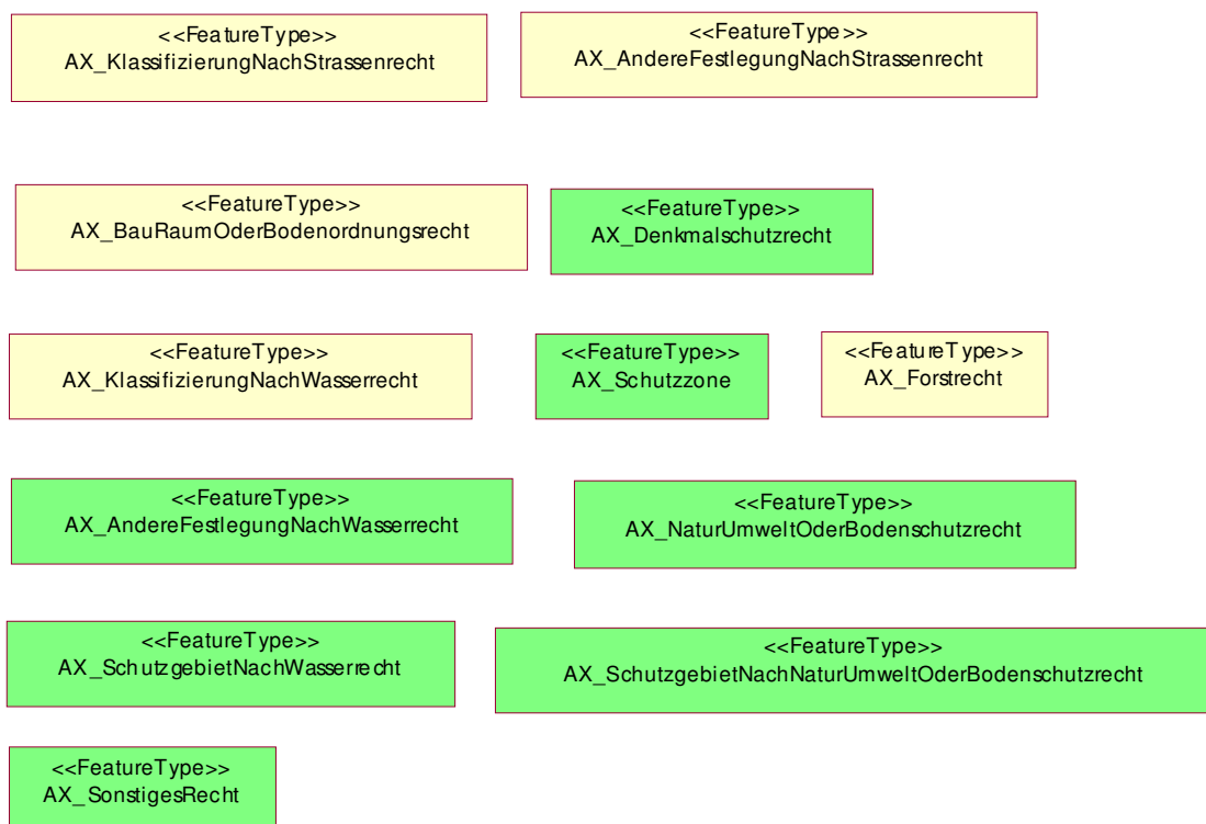
Abbildung 5.4 – 34. : Gesetzliche Festlegungen aus UML
