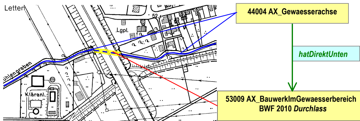
Abbildung 5.4 – 9. : Beispiel für die Modellierung eines Durchlasses
