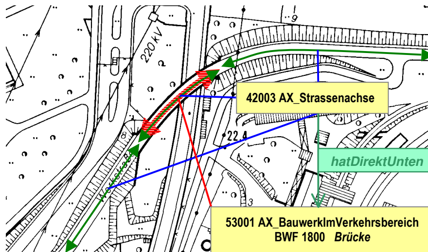
Abbildung 5.4 – 8. : Vertikale Abbildung der Landschaft mit der Relation „hatDirektUnten“
