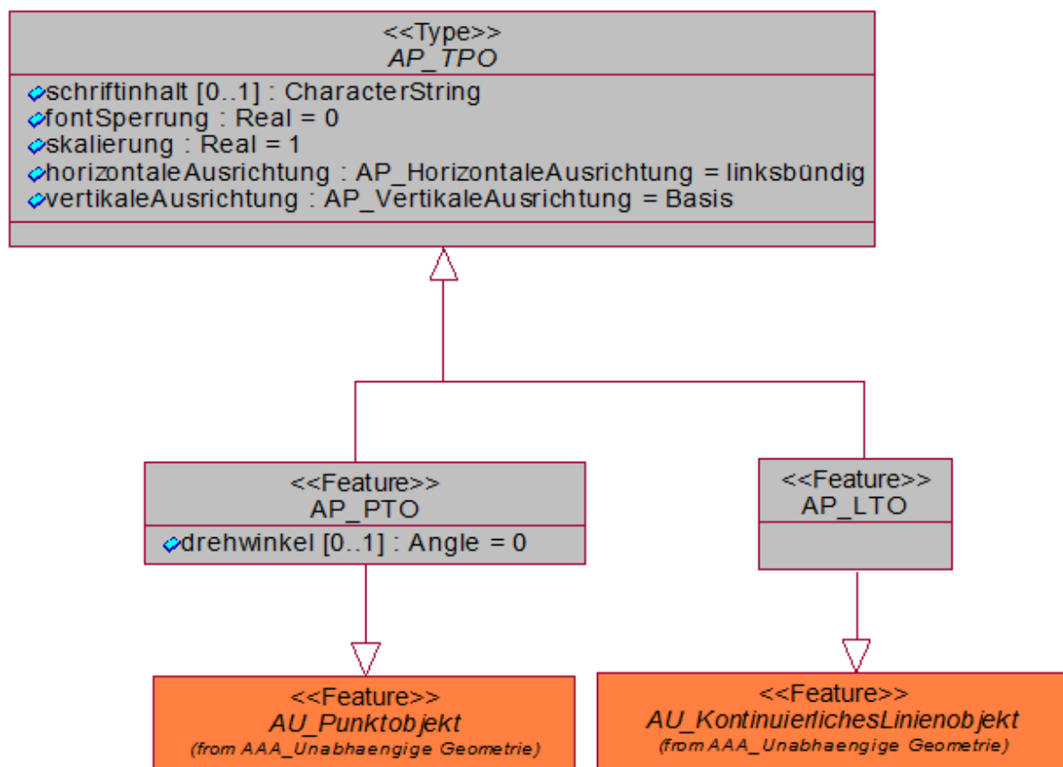
Abbildung 25: Auszug aus Basisschema, AP_TPO
