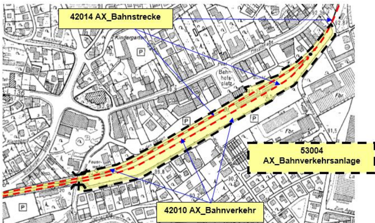
Abbildung 39: Modellierung mehrerer Bahnstrecken
