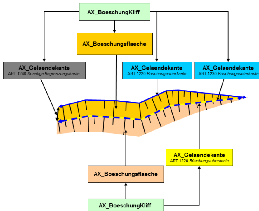
Abbildung 62: Modellierung von Böschungen mit Böschungsflächen und Geländekanten
