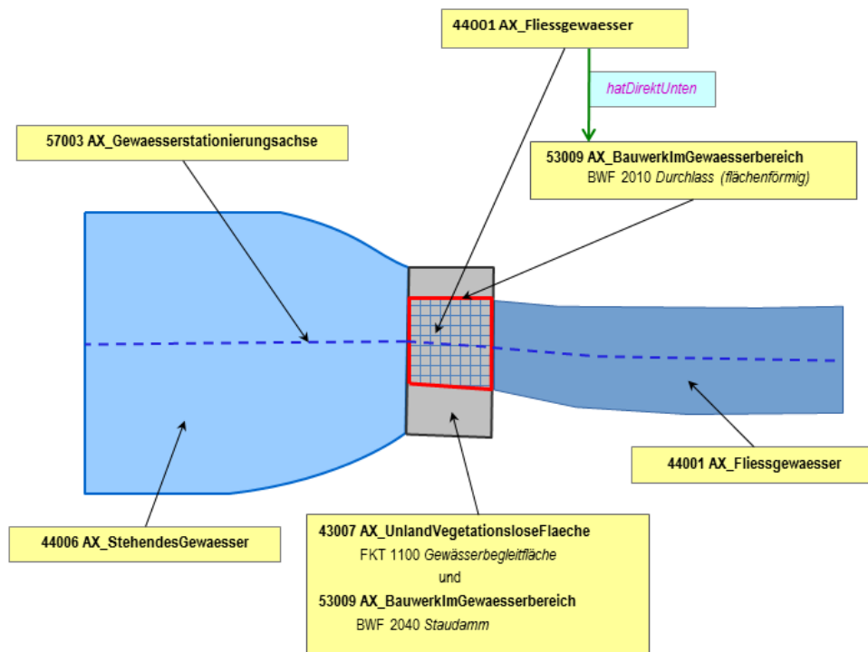
Abbildung 58: Modellierung von Wasserlauf unter Staudamm in flächenförmigem Durchlass Verläuft ein Verkehrsweg wie z. B. eine Straßenachse auf einem Staudamm oder einer Staumauer erhält dieser eine „hatDirektUnten“-Relation zum Bauwerk. Dadurch wird die Grundfläche, auf der das Bauwerk liegt, nicht geteilt.
