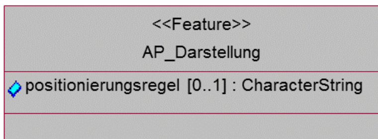
Abbildung 24. Auszug aus Basisschema, AP_Darstellung
