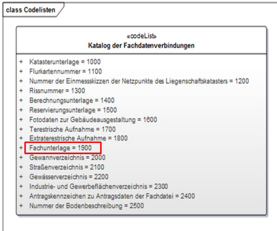
Abbildung 3: Codeliste „Katalog der Fachdatenverbindungen“
