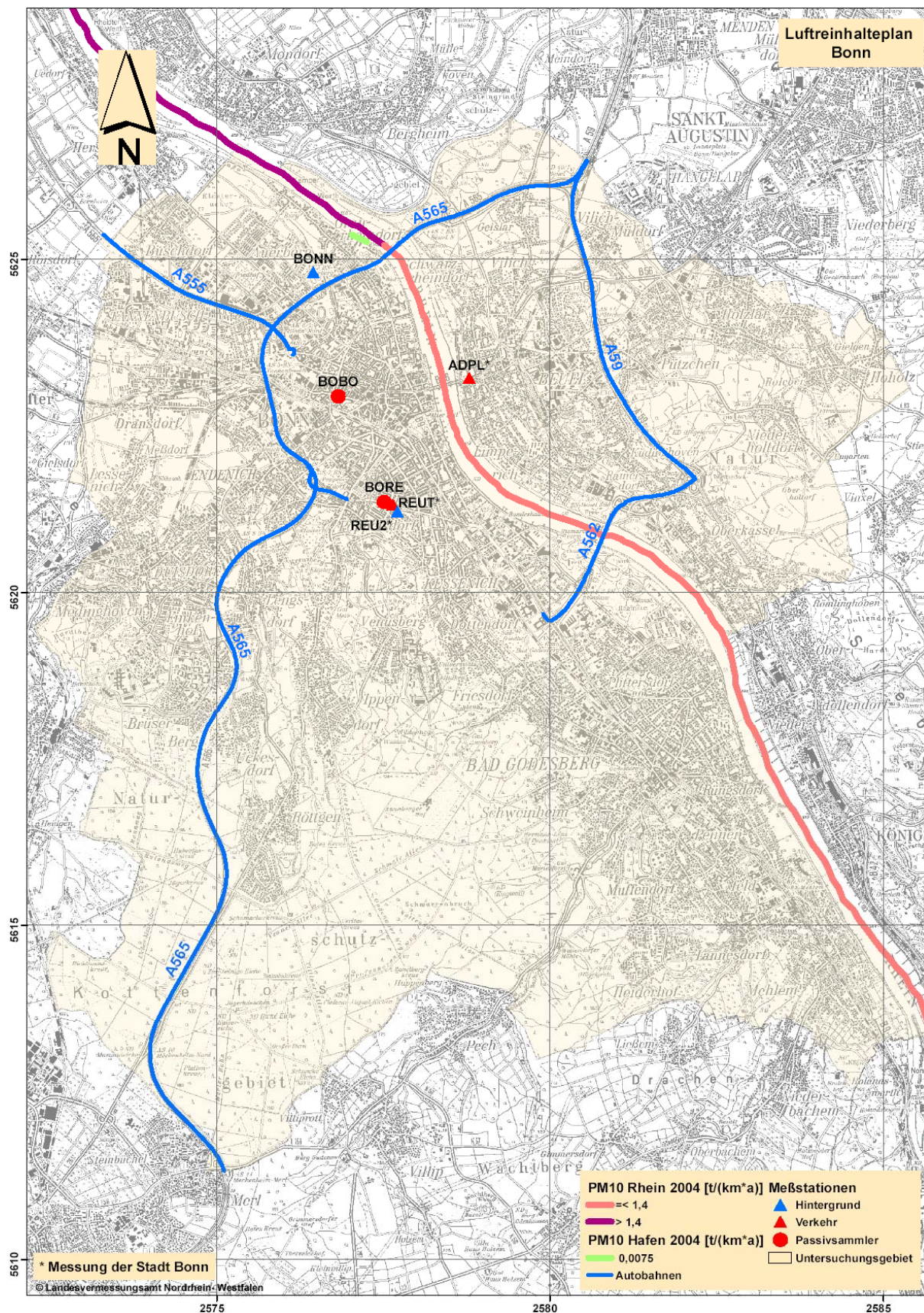
Abb. 3.2/7: \text{PM}_{10} -Emissionen des Schiffsverkehrs im Untersuchungsgebiet (2004)
