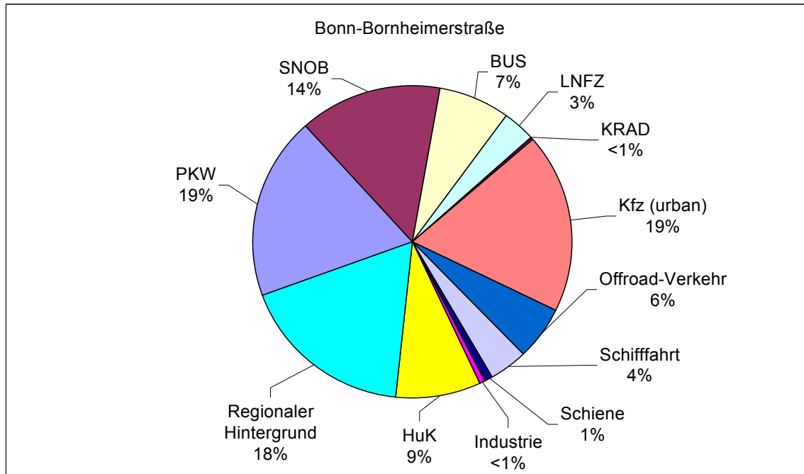
Abb. 3.3/2: Darstellung der berechneten prozentualen Beiträge der verschiedenen Verursachergruppen sowie des regionalen Hintergrundniveaus an der \text{NO}_x -Belastung an der Messstelle Bornheimer Straße (BOBO)
