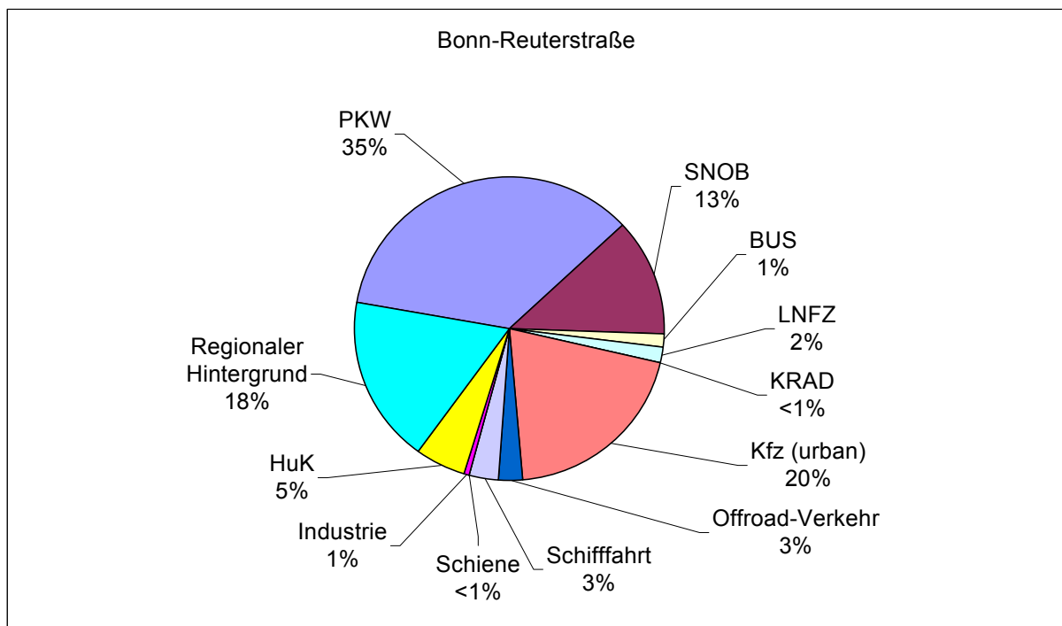
Abb. 4.2/3: Darstellung der berechneten prozentualen Beiträge der verschiedenen Verursachergruppen sowie des regionalen Hintergrundniveaus an der NO x -Belastung für das Zieljahr 2010 an der Reuterstraße (BORE)
