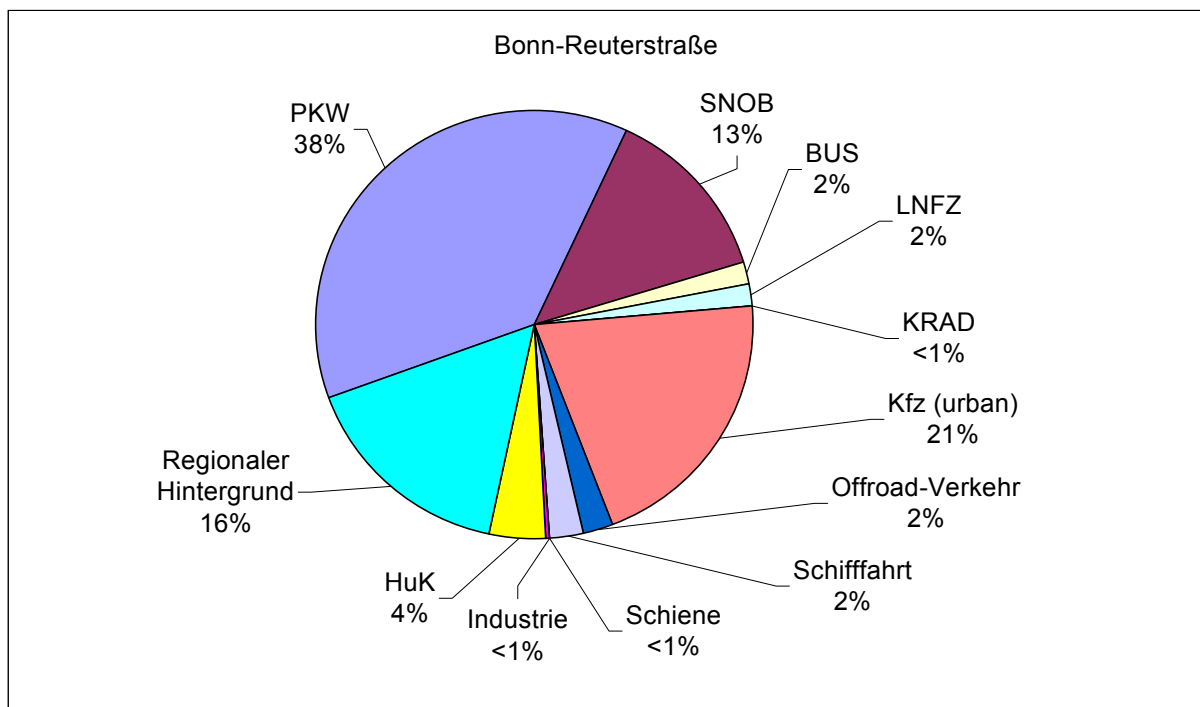
Abb. 3.3/3: Darstellung der berechneten prozentualen Beiträge der verschiedenen Verursachergruppen sowie des regionalen Hintergrundniveaus an der NO x -Belastung an der Messstelle Bonn-Reuterstraße (BORE)
