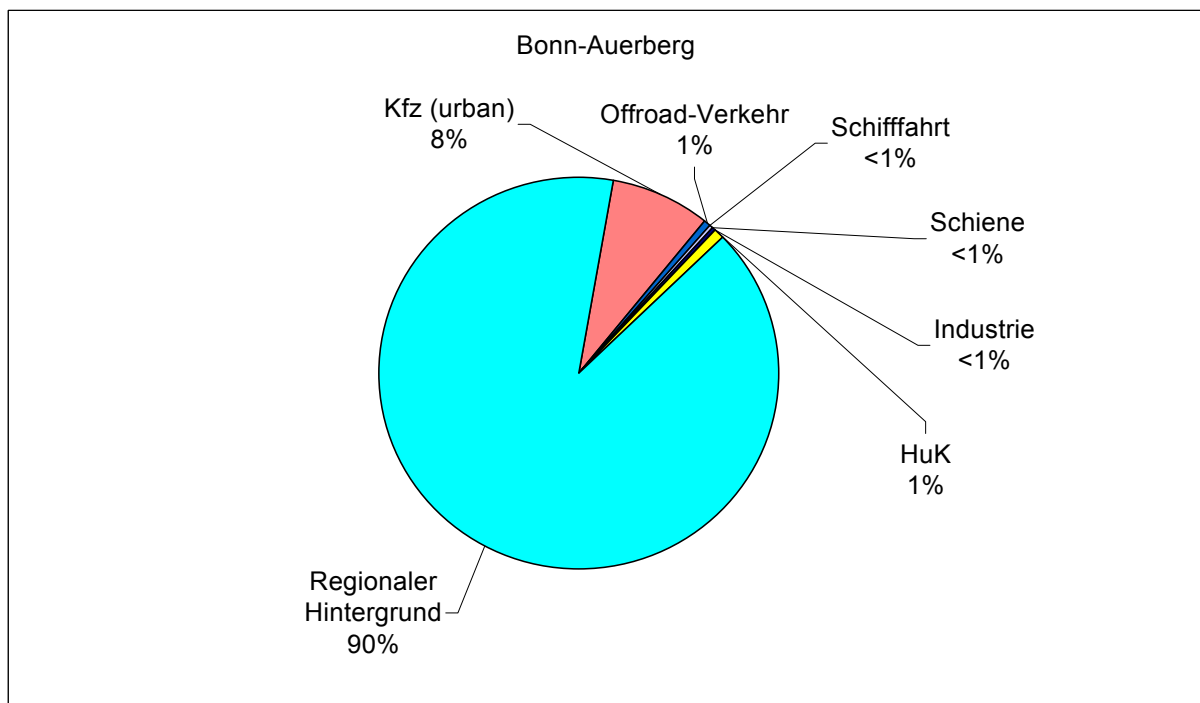
Abb. 3.3/4: Darstellung der berechneten prozentualen Beiträge der verschiedenen Verursachergruppen sowie des regionalen Hintergrundniveaus an der PM 10 -Belastung an der Messstelle Bonn-Auerberg (BONN)
