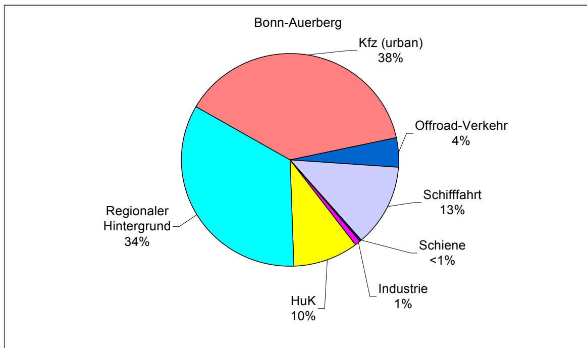
Abb. 3.3/1: Darstellung der berechneten prozentualen Beiträge der verschiedenen Verursachergruppen sowie des regionalen Hintergrundniveaus an der \text{NO}_x -Belastung an der Messstelle Bonn-Auerberg (BONN)
