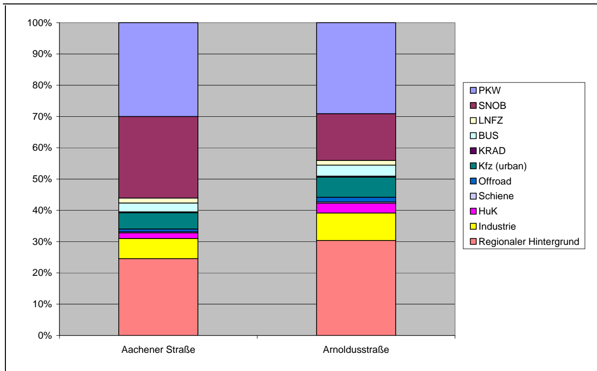
Abb. 4.2/3: Darstellung der prozentual berechneten Beiträge der Verursachergruppen sowie des regionalen Hintergrunds für die NO x -Belastung im Prognosejahr 2015 an den Verdachtsfällen mit berechneter Grenzwertüberschreitung
