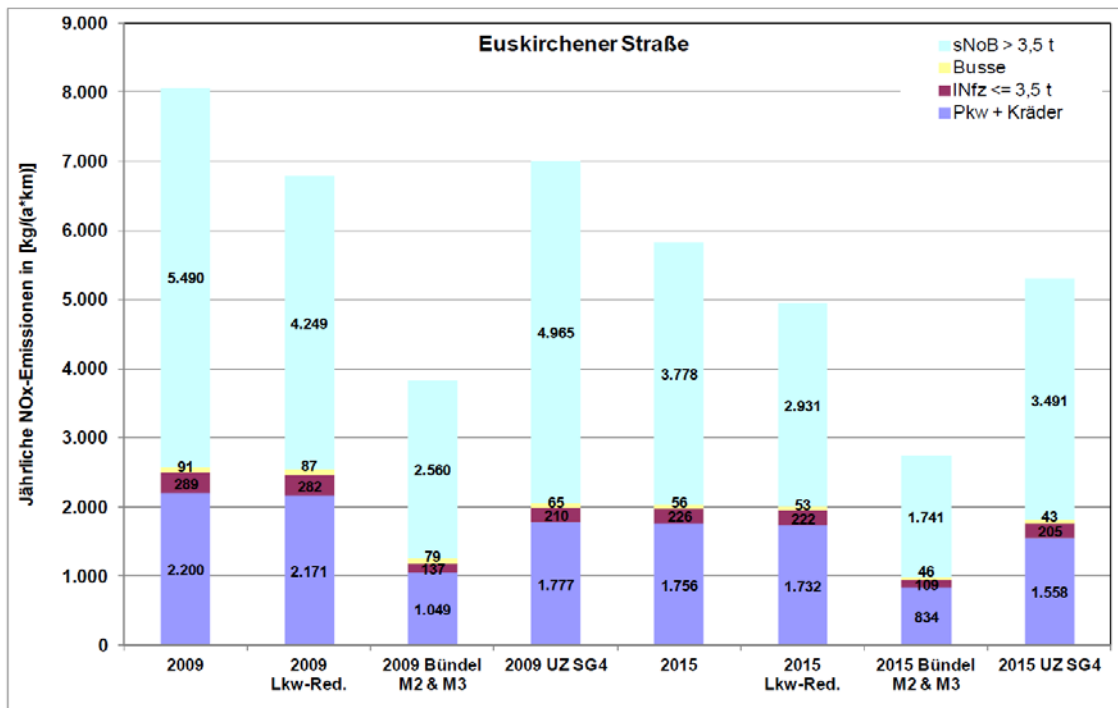
Abb 6.2/1: NO x -Emissionsanteile verschiedener Fahrzeugarten am Hot Spot Euskirchener Straße im Analysejahr 2009 sowie im Prognosejahr 2015 ohne und mit den Maßnahmen:
